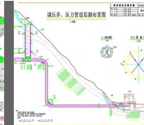
熊貓水電站壓力管道監測佈置圖
