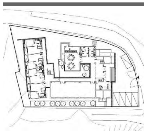
三江保護站 平面圖
