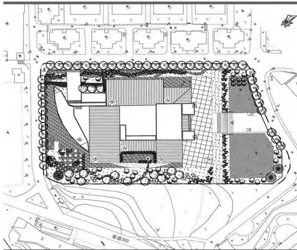
總平面圖
