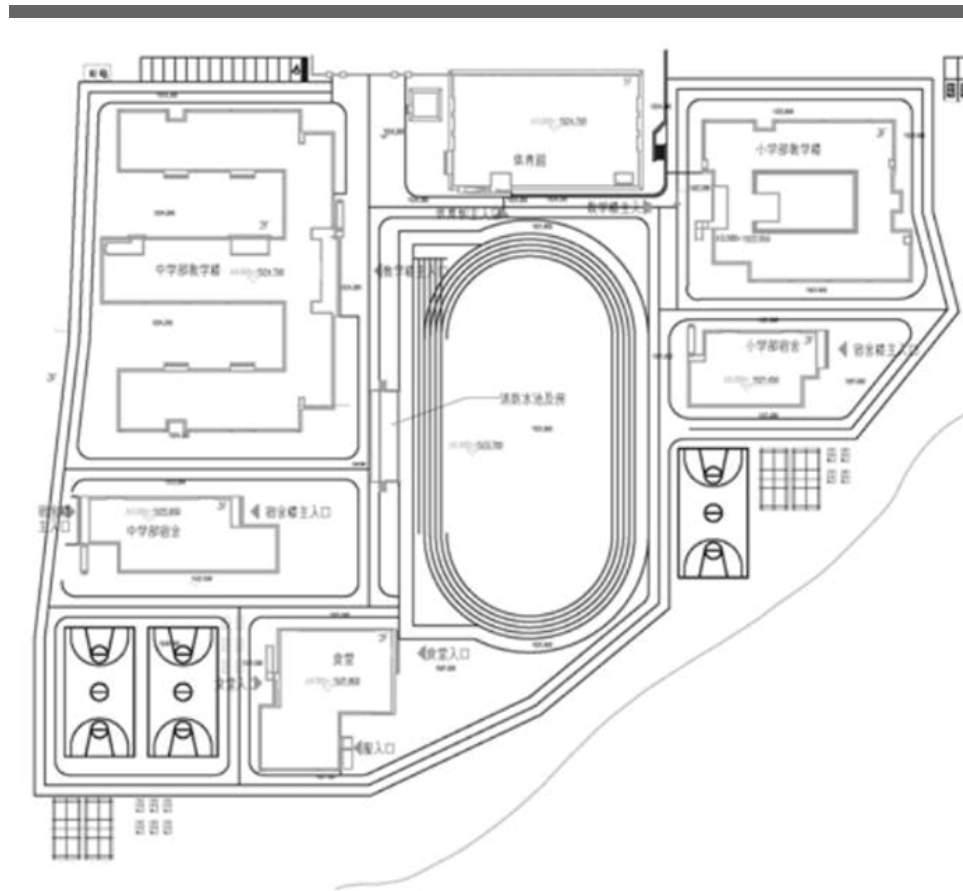
平面圖
